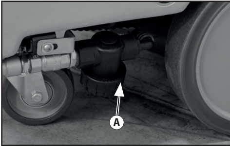
Foto 24 A) Reinigungslösungsfilter
